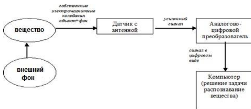
Рис. 2. Структурная схема системы распознавания веществ.
